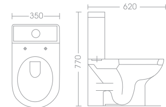
DOBRA W.C. TOILET 71-6315 62 X 35 X 77 White
