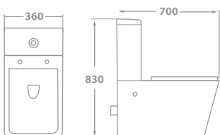
KING W.C. TOILET 71-6200 70 X 36 X 83 White
