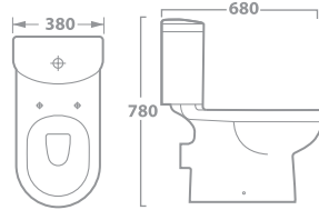
SOFIA W.C. TOILET 71-6050 68 X 38 X 78 White 71-6051 68 X 38 X 78 Ivory
