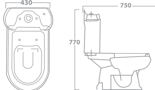
MAGNOM W.C. TOILET 71-1101 75 X 43 X 77 White 71-1111 75 X 43 X 77 Ivory
