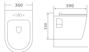
RIGA WALL HUNG TOILET 71-6450 59 X 36 X 33 White 71-6451 59 X 36 X 33 Ivory
