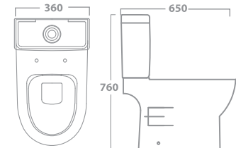
MED W.C. TOILET 71-6140 65 X 36 X 76 White Bottom Inlet 71-6145 65 X 36 X 76 White Side Inlet
