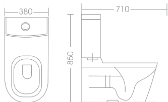
DOME W.C TOILET 71-6330 71 X 38 X 85 White
