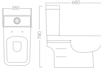
MED W.C. TOILET 71-6190 68 X 38 X 78 White
