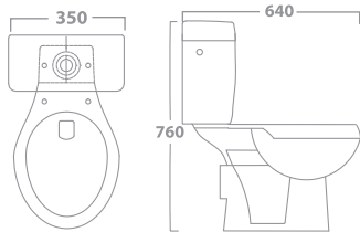
MED W.C. TOILET 71-6120 64 X 35 X 76 White Bottom Inlet 71-6125 64 X 35 X 76 White Side Inlet
