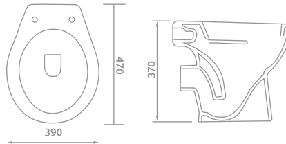
VITRA W.C TOILET 71-6630 47 X 39 X 37 White 71-6631 47 X 39 X 37 Ivory
