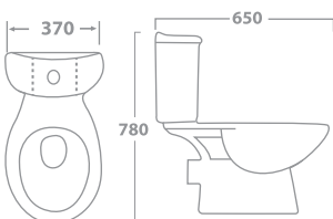
ROGER W.C. TOILET 71-6150 65 X 37 X 78 White 71-6151 65 X 37 X 78 Ivory
