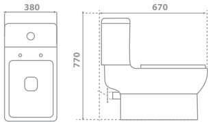
MAGIC W.C. TOILET 71-1061 67 X 38 X 77 White 71-1071 67 X 38 X 77 Ivory
